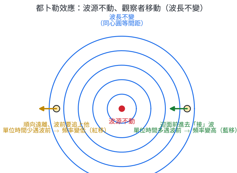
圖 4-7：波源不動、觀察者移動。波源發出的是一圈圈等間距的同心圓（波長不變）；迎面前進的觀察者單位時間遇到較多波前（頻率變高、藍移），順向遠離的觀察者單位時間遇到較少波前（頻率變低、紅移）。
